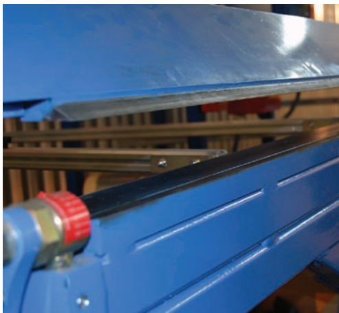
Гибочная балка станка-аналога
